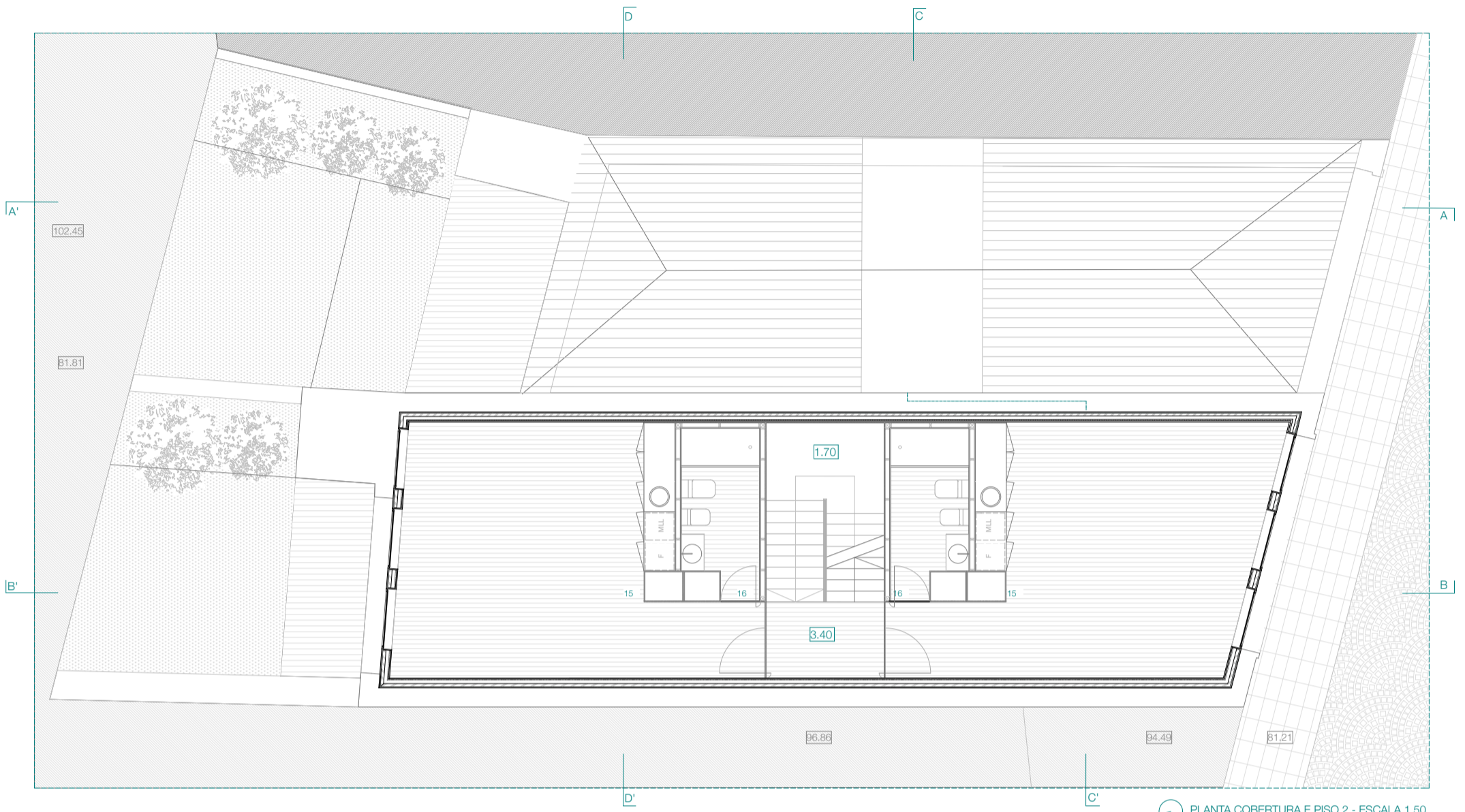
PLANTA COBERTURA E PISO 2 - ESCALA 1.50
