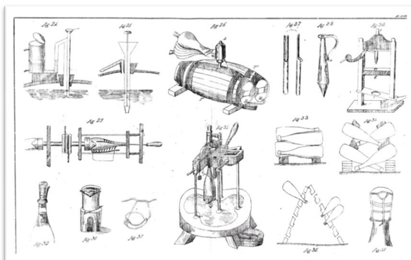
Ilustração 102 - Tecnologia Agrícola de Ferreira Lapa
