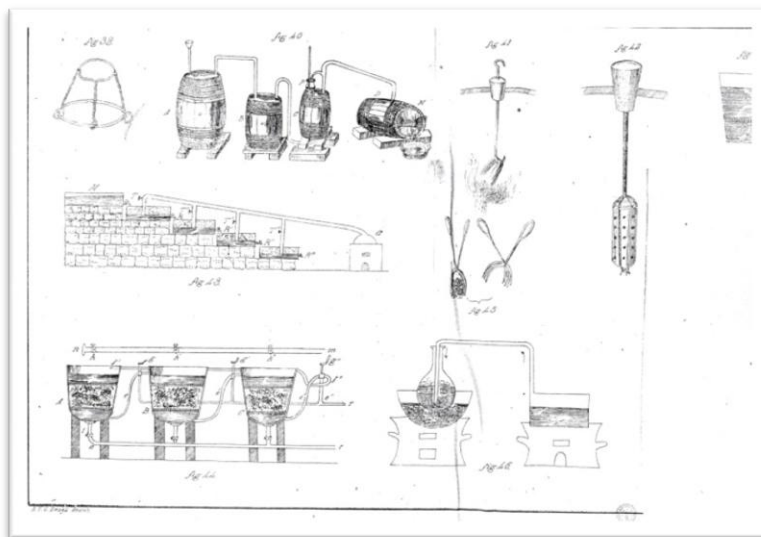
Ilustração 85 – Tecnologia Agrícola de Ferreira Lapa
