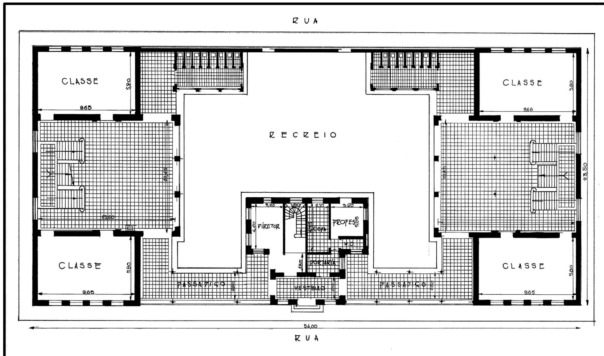
Figura 50- Estudo elaborado pelo autor sobre planta de 1912. Planta baixa do pavimento térreo dos edifícios Escola de Meninas e Escola de Meninos.
