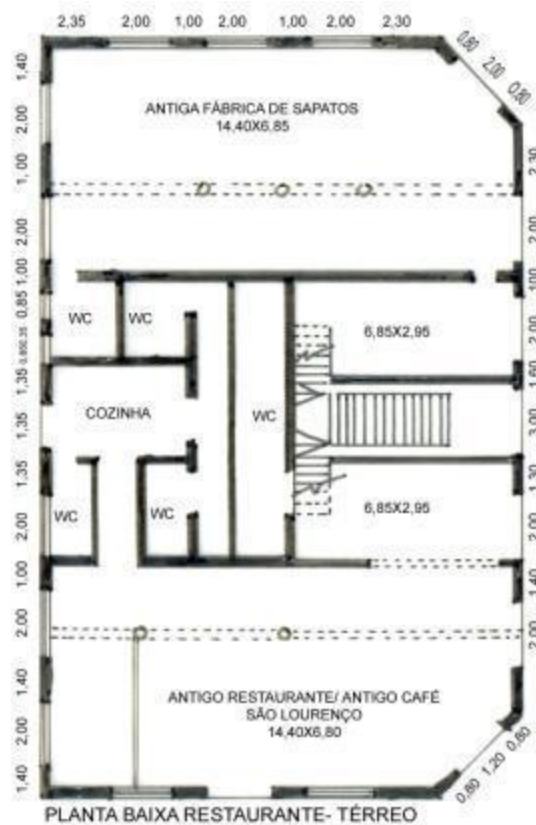
Figura 59- - Estudo elaborado pelo autor sobre projeto de Luiz Magnani. Planta baixa do restaurante- o térreo.
