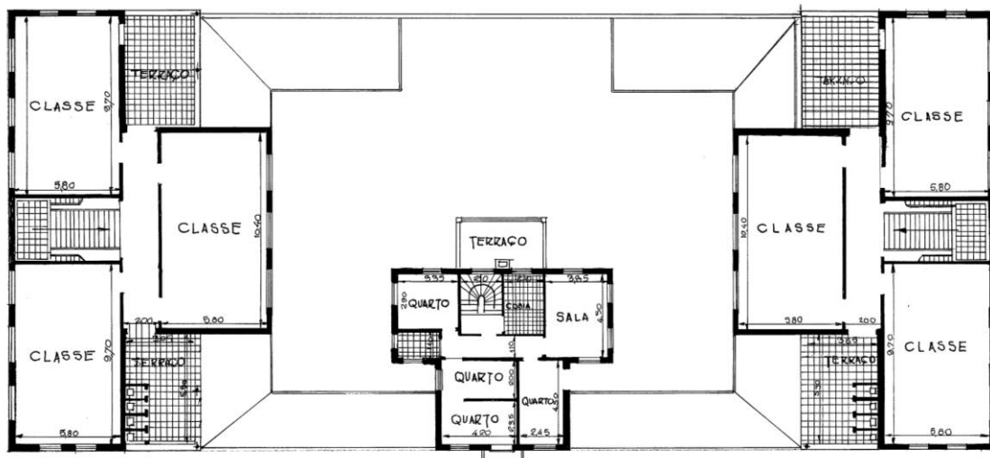
Figura 87-Planta original do primeiro andar das Escolas dos Meninos e Meninas
