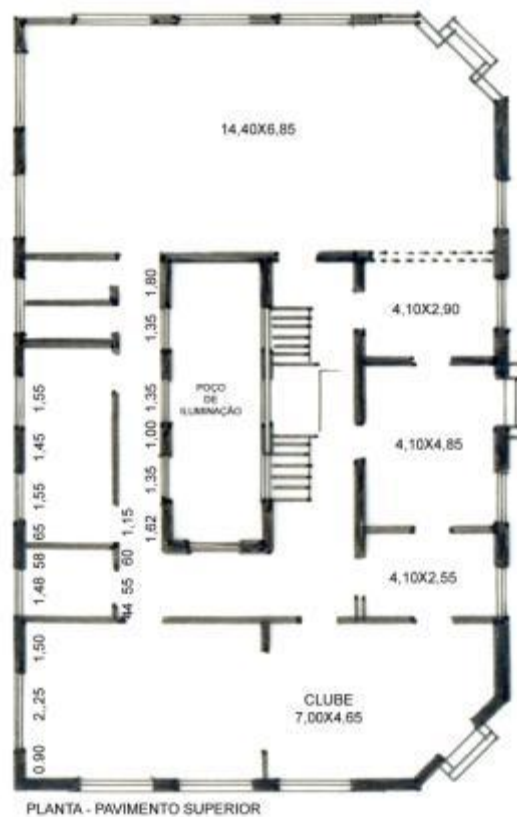
Figura 60- - Estudo elaborado pelo autor sobre projeto de Luiz Magnani. Planta do restaurante, primeiro pavimento.
