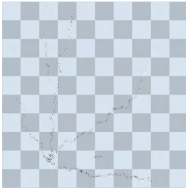
(d) Step 4000
