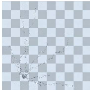
(j) Step 10000
