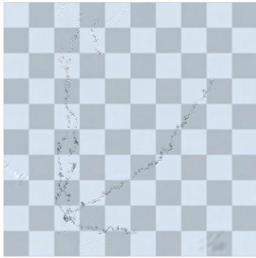
(d) Step 4000
