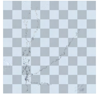
(f) Step 6000
