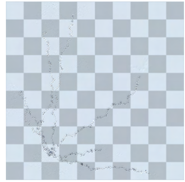
(f) Step 6000
