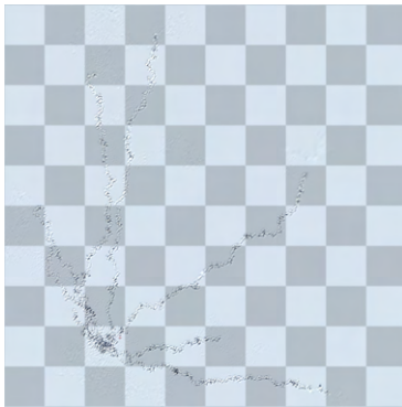
(g) Step 7000
