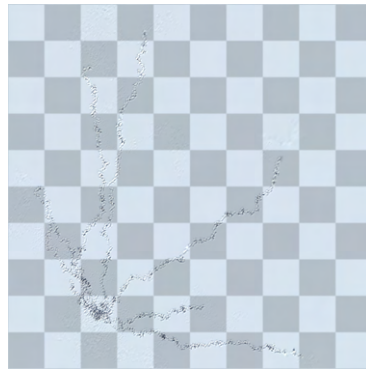
(h) Step 8000
