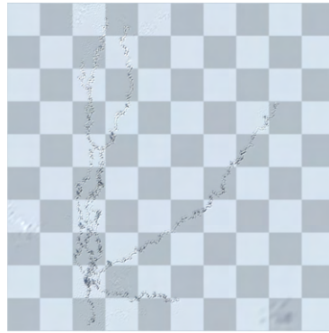
(e) Step 5000
