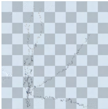
(g) Step 7000
